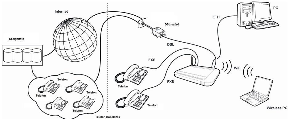
1. ábra: Hálózati példa (VoIP szolgáltatás esetén)
