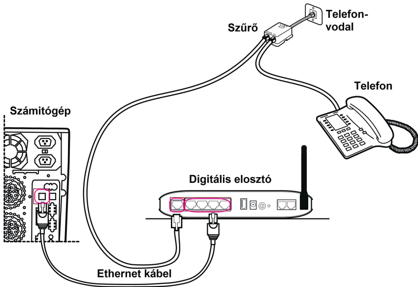
5. ábra: Az Ethernet kábel csatlakoztatása
