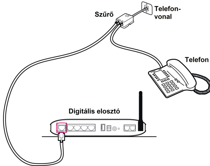
6. ábra: A telefonok csatlakoztatása
