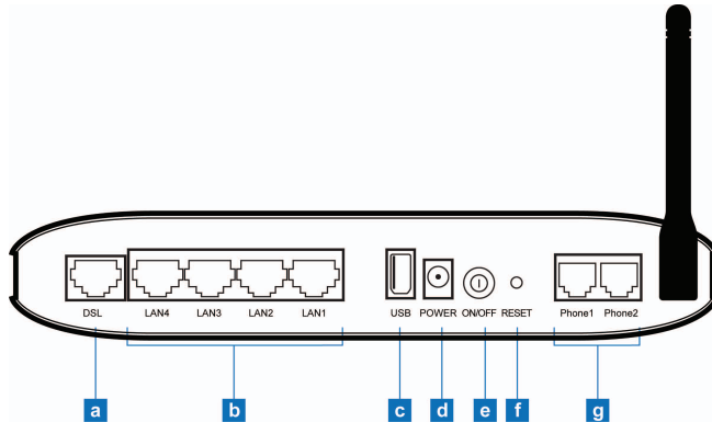
3. ábra: A digitális elosztó hátlapja
