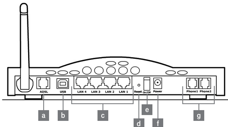
3. ábra: A digitális elosztó hátlapja
